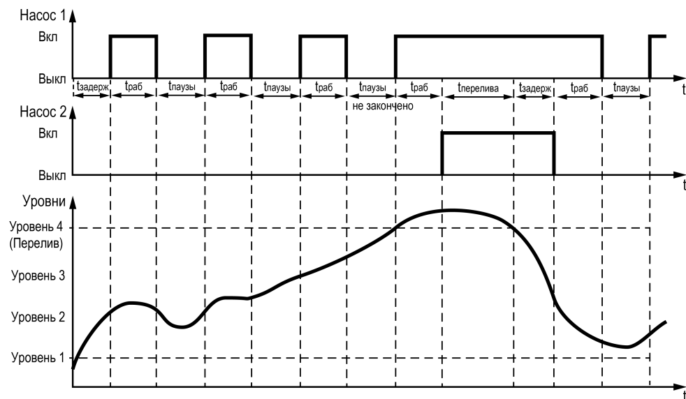
Рисунок 9.6 – Авария аналогового датчика уровня
