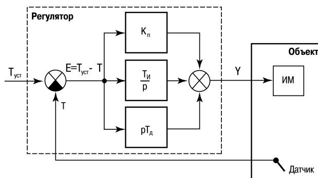
Рисунок 7.7 – Структурная схема ПИД-регулятора
