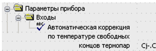
Рисунок 10.4 – Параметр Автоматическая коррекция показаний прибора по температуре свободных концов термопар (Сj-.C)
