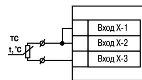
Рисунок 5.5 – Двухпроводная схема подключения ТС
