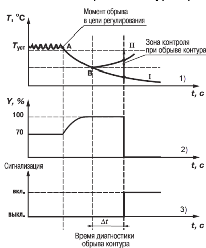
Рисунок 7.17 – Срабатывание диагностики обрыва
