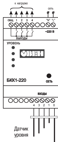
Рисунок 5.4 – Схема подключения БКК1-220
