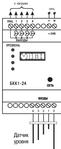
Рисунок 5.3 – Схема подключения БКК1-24
